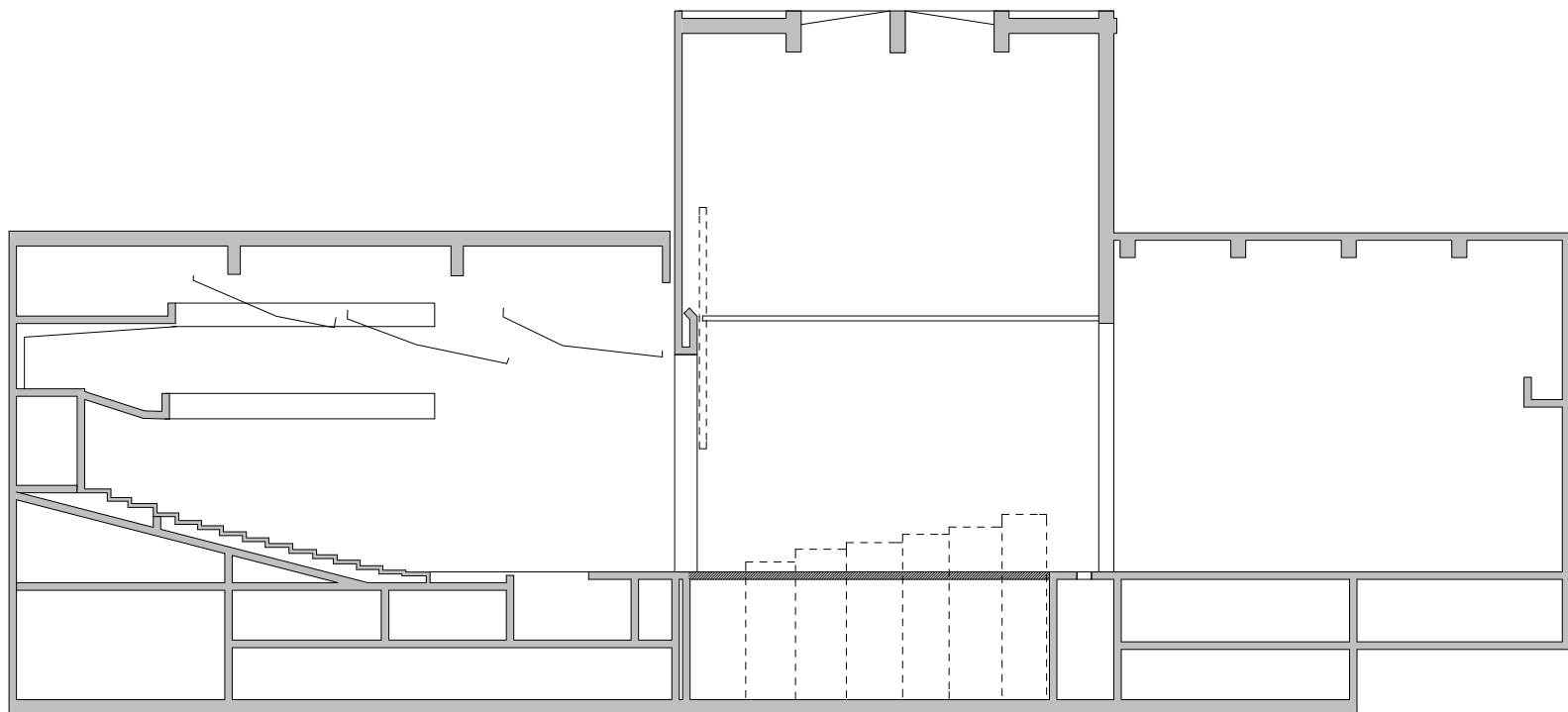
Srpsko narodno pozorište, Novi sad presek velike sale R 1:300
