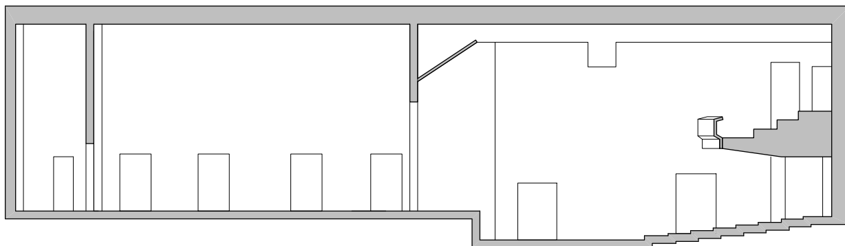
Kruševačko pozorište presek R 1:200
