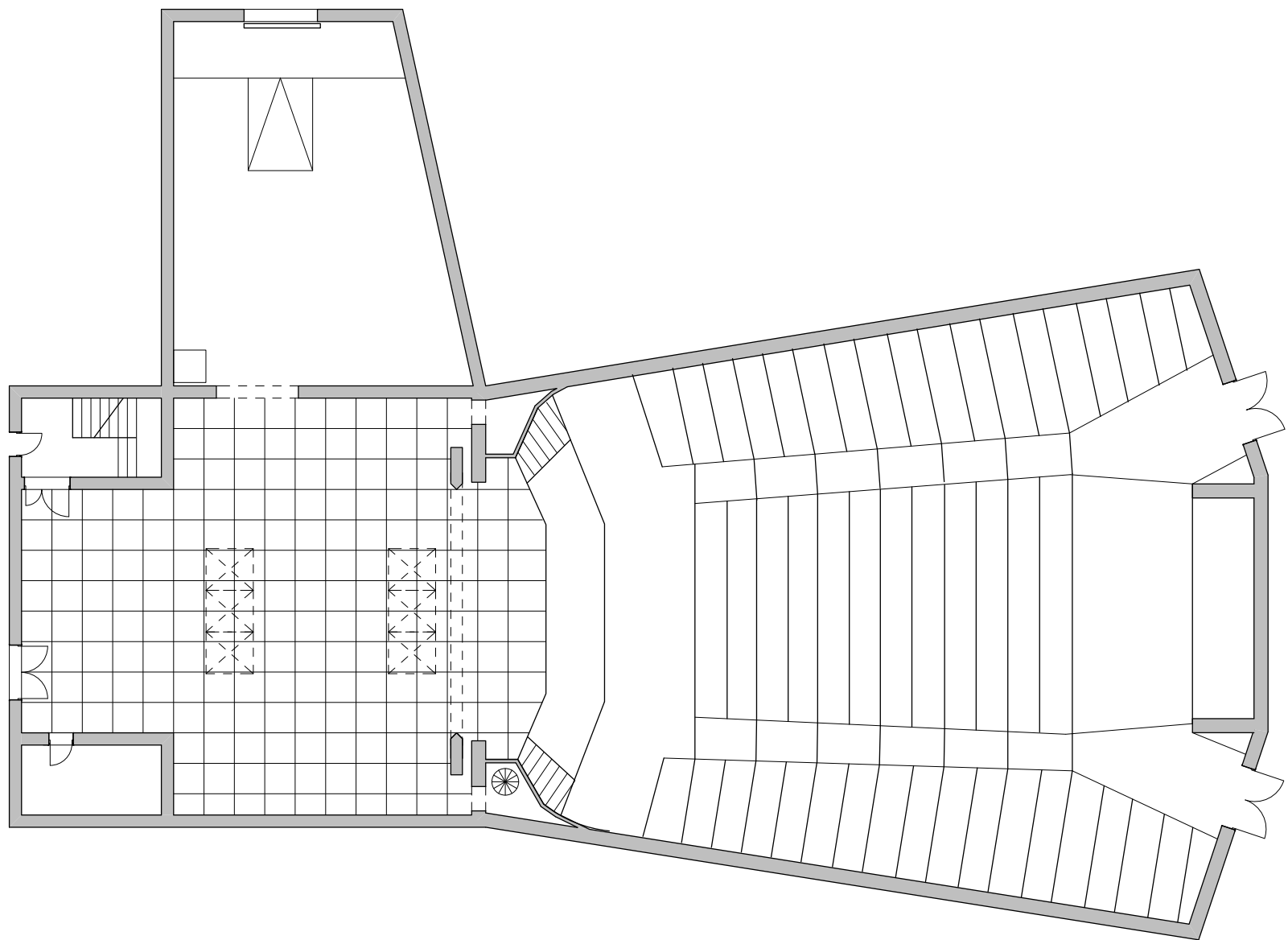
Pozorište u Užicu osnova velike sale R 1:200
