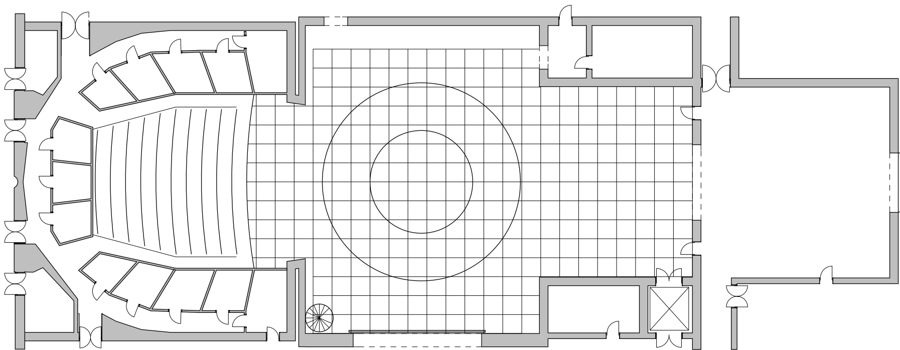
Narodno pozorište u Sombor osnova R 1:200
