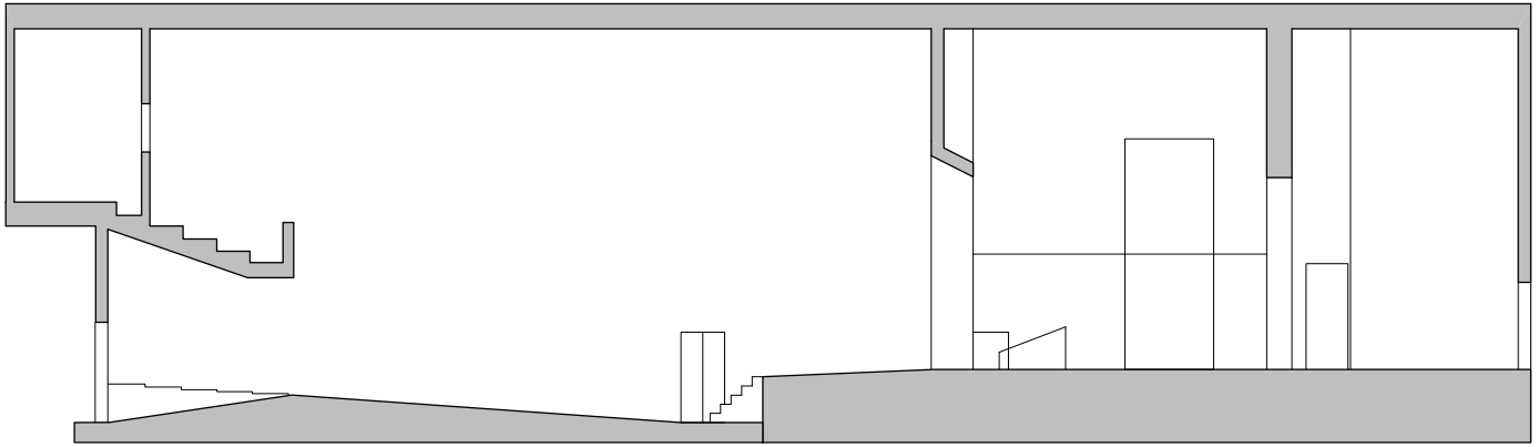
Pozorište mladih, Novi Sad presek velike sale R 1:200
