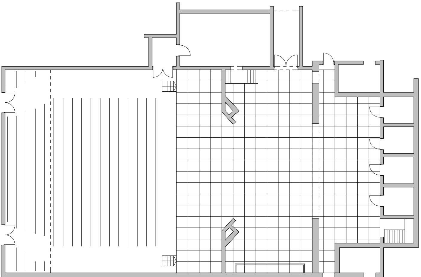
Pozorište mladih, Novi Sad osnova velike sale R 1:200
