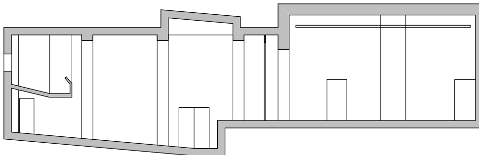
Novosadsko pozorište - Újvidéki Színház presek velike sale R 1:200
