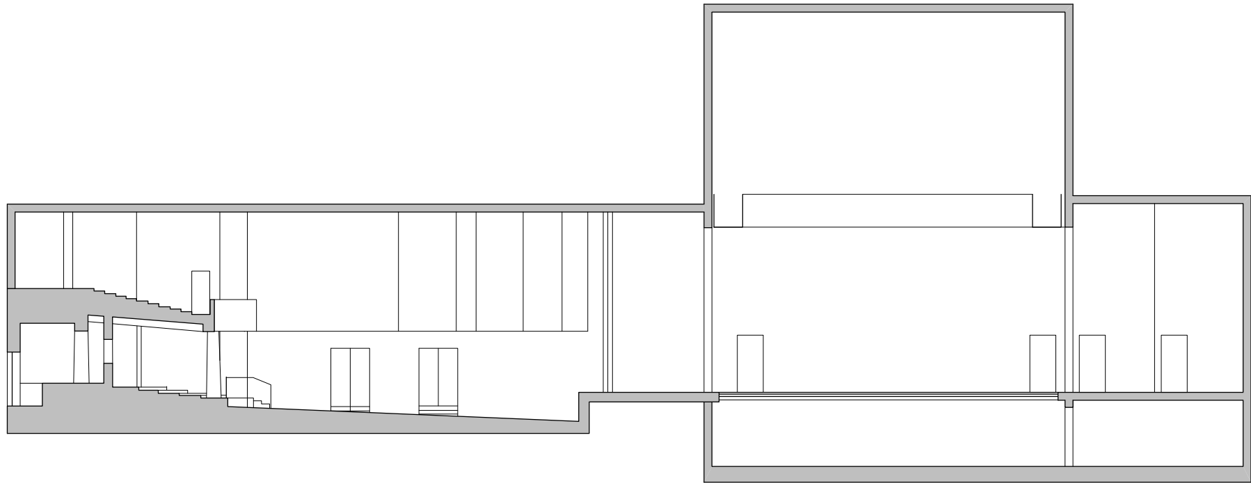
Pozorište u Šapcu presek R 1:200
