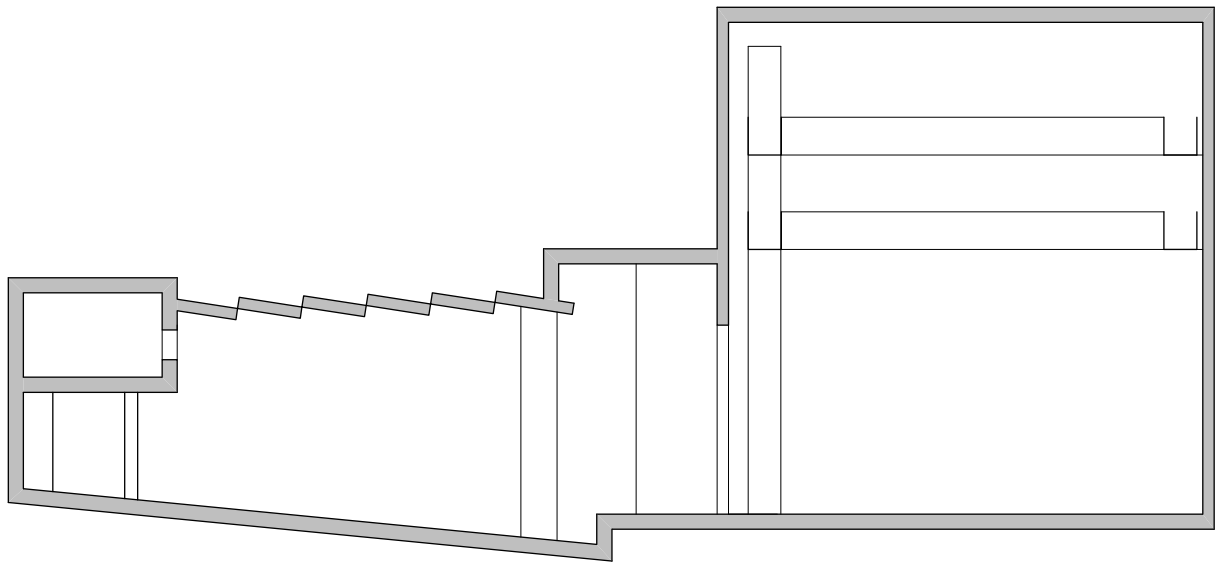
Pozorište u Zaječaru presek R 1:200
