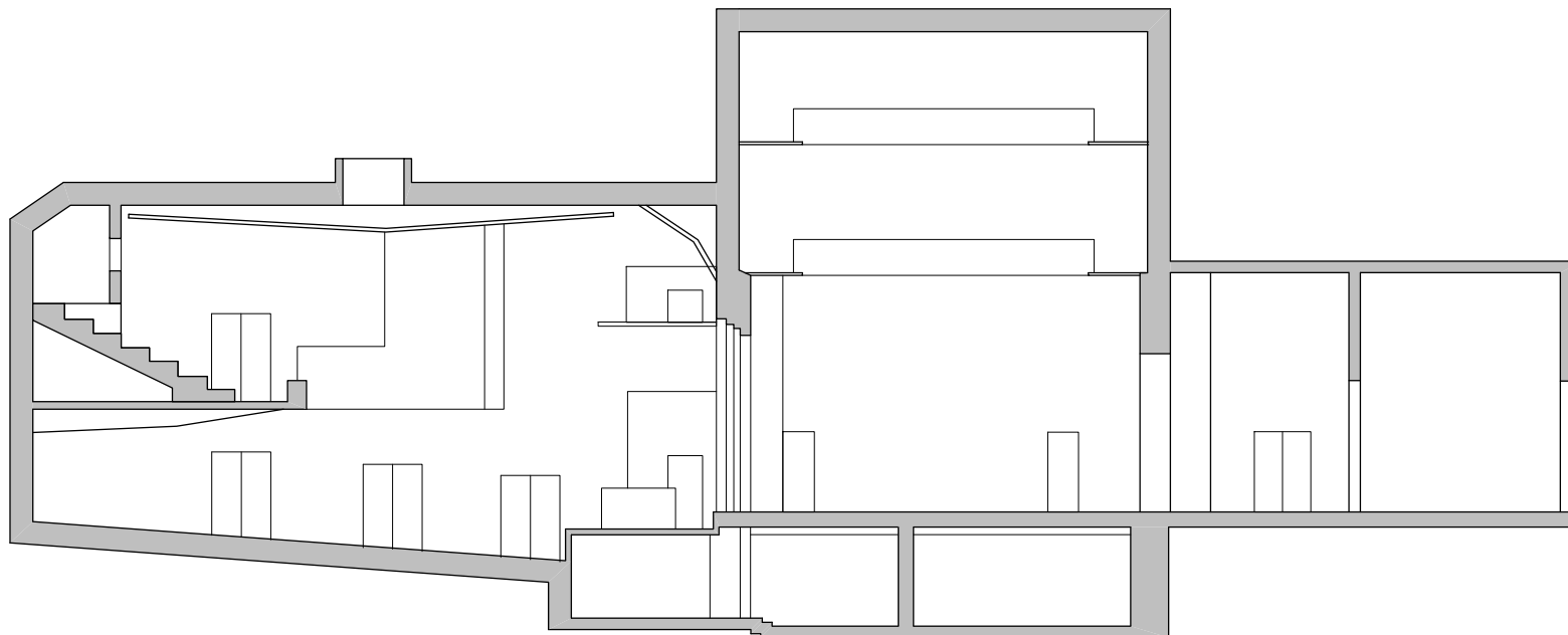
Narodno pozorište u Nišu presek R 1:200
