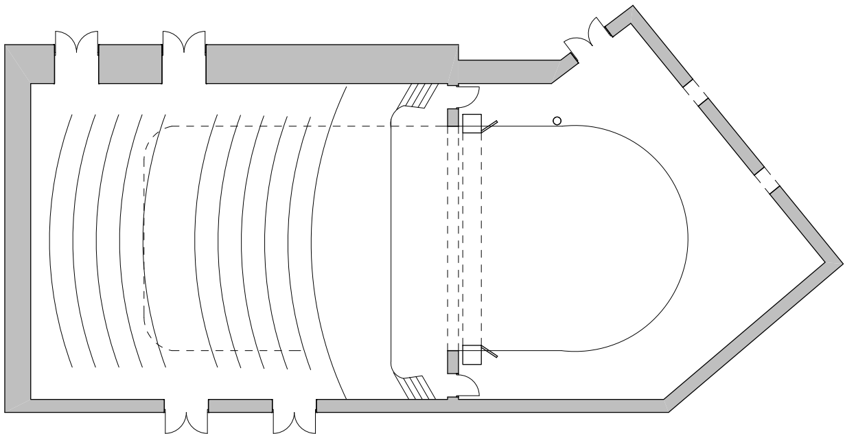
Pozorište u Sremskoj Mitrovici osnova R 1:200
