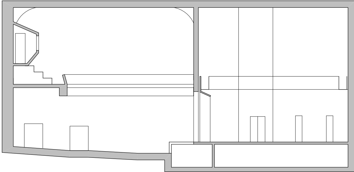
Pozorište u Sremskoj Mitrovici presek R 1:200
