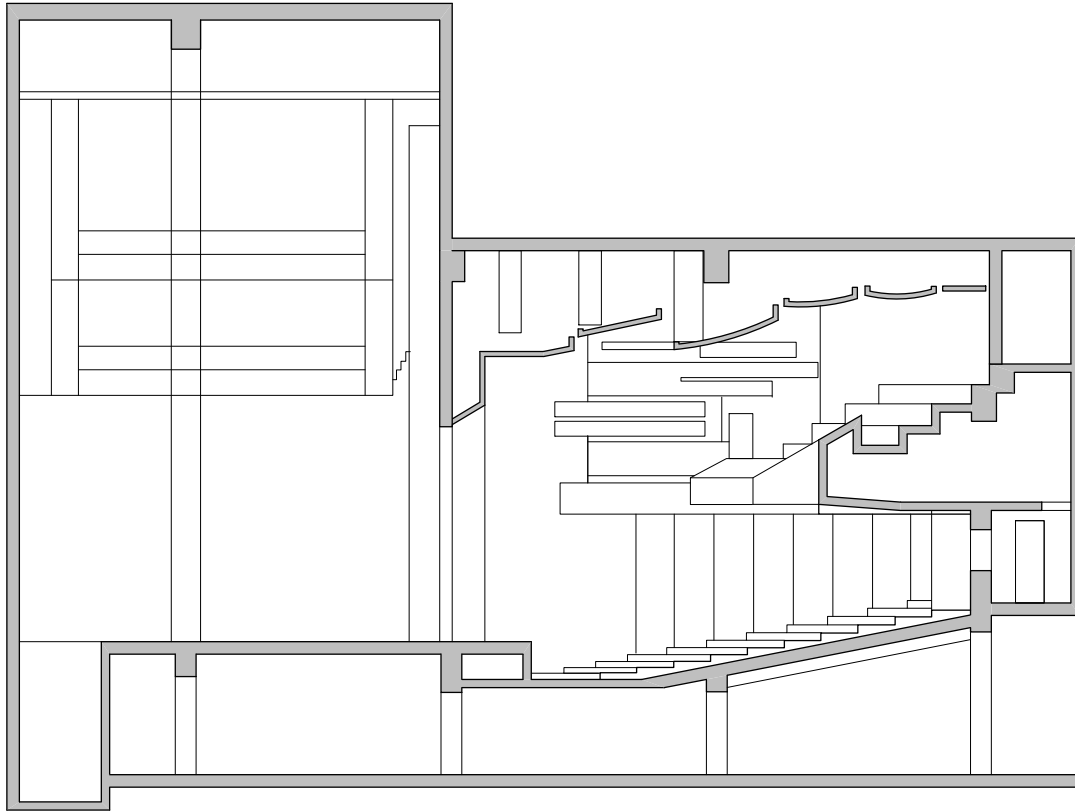
Pozorišna sala NIS-a, Novi Sad presek R 1:200
