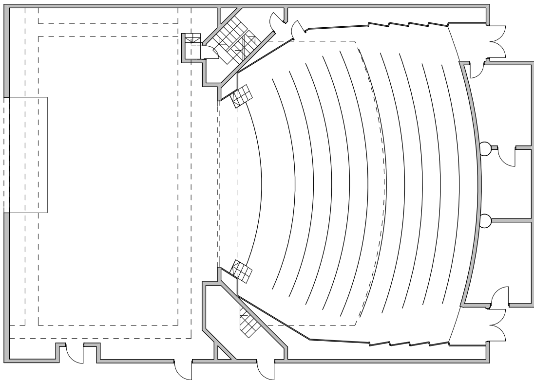
Pozorišna sala NIS-a, Novi Sad osnova R 1:200
