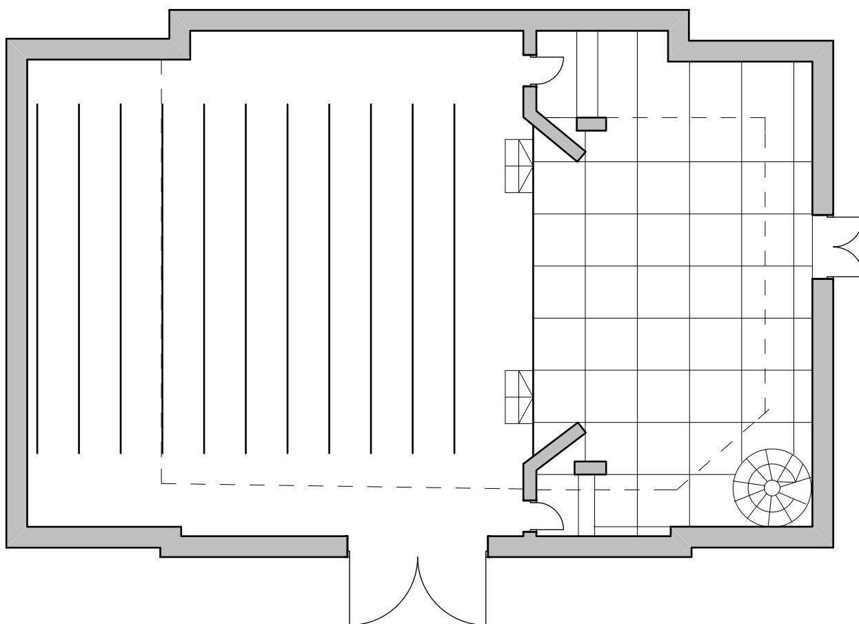
Pozorište mladih, Novi Sad osnova male sale R 1:100
