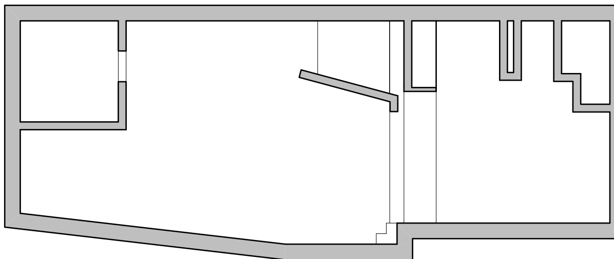
Pozorište mladih, Novi Sad presek male sale R 1:100
