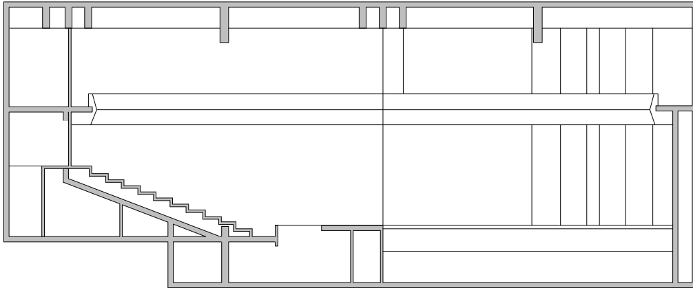
Srpsko narodno pozorište, Novi sad presek male sale R 1:300
