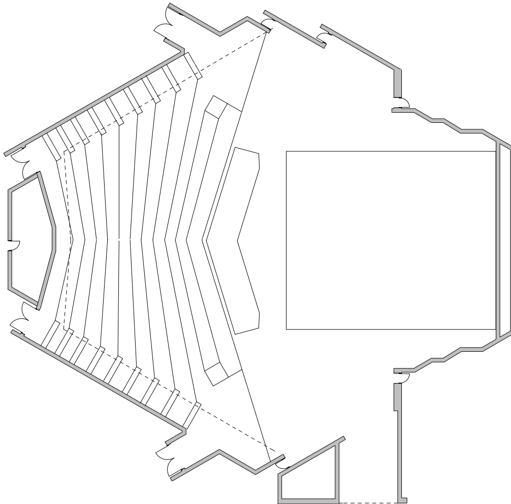
Srpsko narodno pozorište, Novi sad osnova male sale R 1:300
