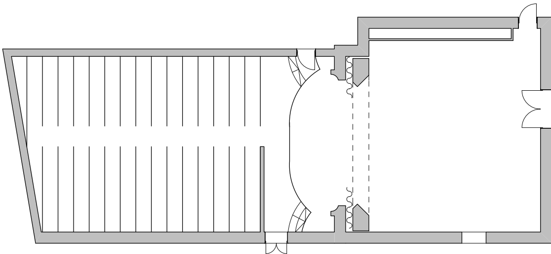
Pozorište u Kraljevu osnova R 1:200
