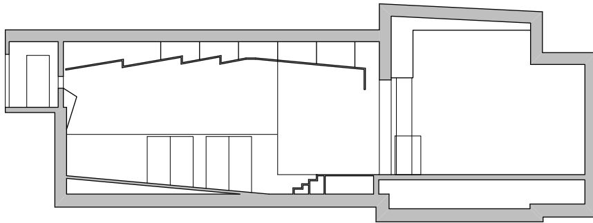
Dečije pozorište u Subotici presek R 1:200
