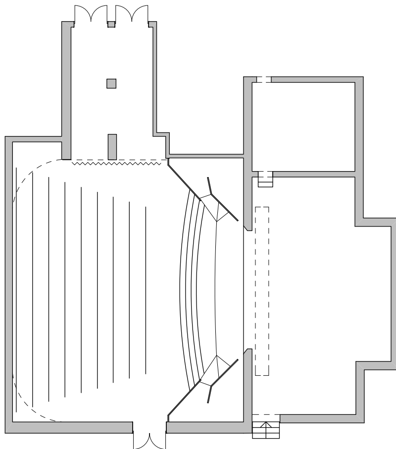
Dečije pozorište u Subotici osnova R 1:200
