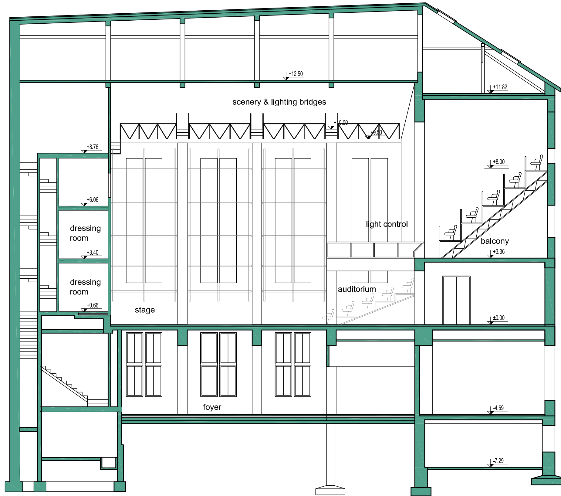
longitudinal section
