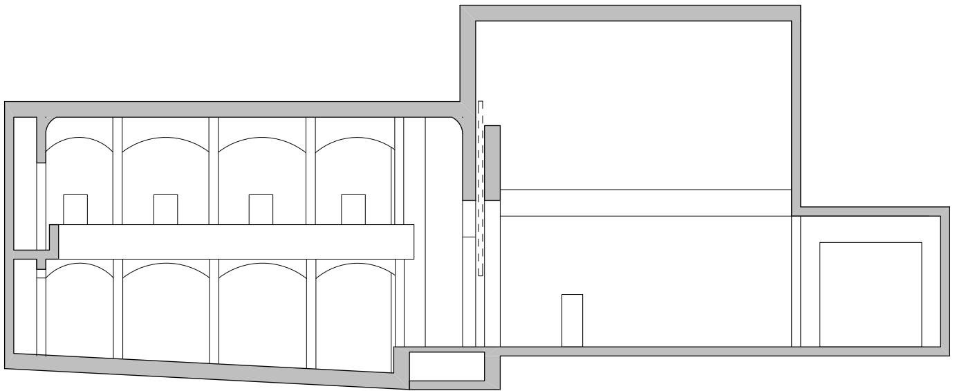
Narodno pozorište „Sterija”, Vršac presek R 1:200
