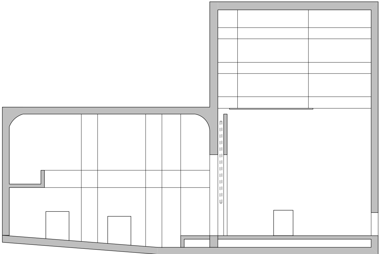
Narodno pozorište Kikinda presek R 1:200
