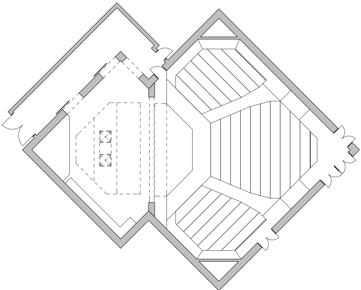
Pozorište „Duško Radović“, Beogra osnova R 1:200
