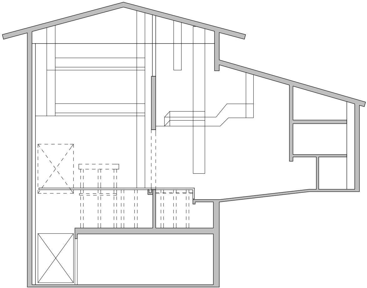
Pozorište „Duško Radović“, Beograd presek R 1:200
