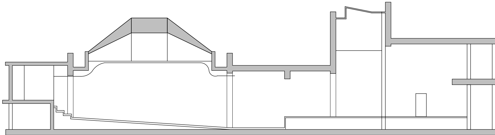
Pozorište „Boško Buha“, Beograd presek R 1:200
