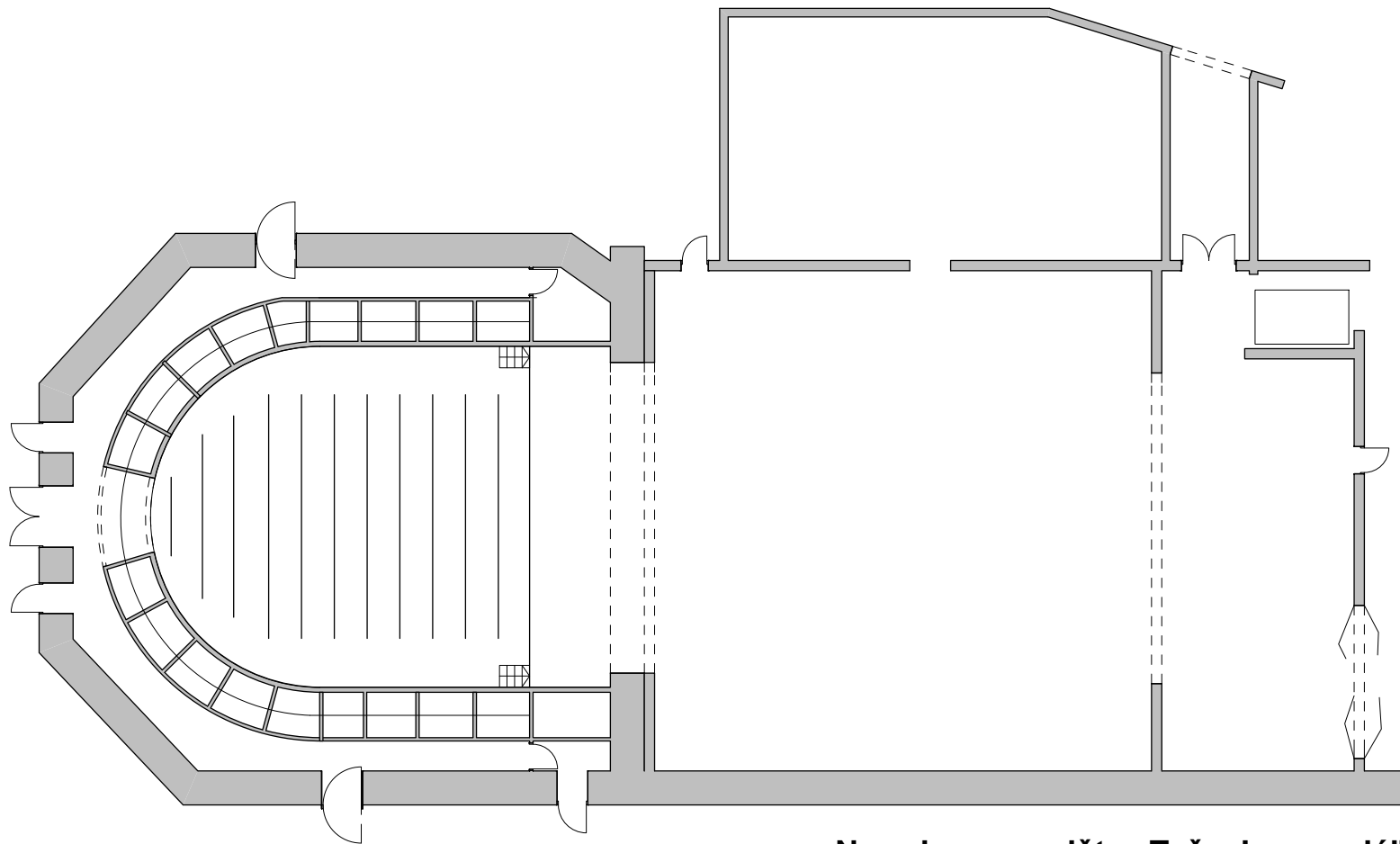
Narodno pozorište „Toša Jovanović” osnova R 1:200
