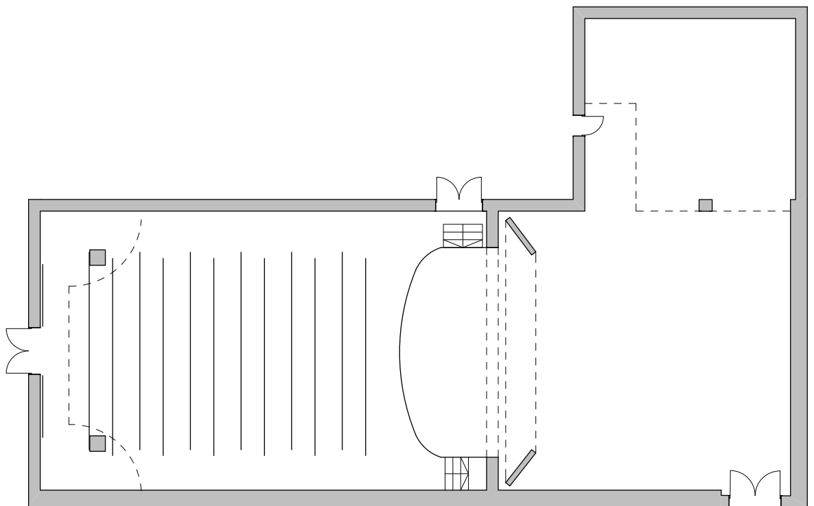
Pozorište u Vranju osnova R 1:200
