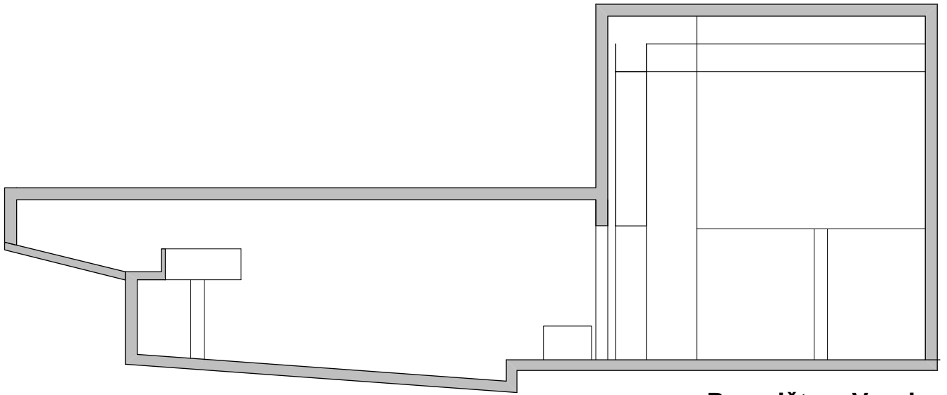
Pozorište u Vranju presek R 1:200
