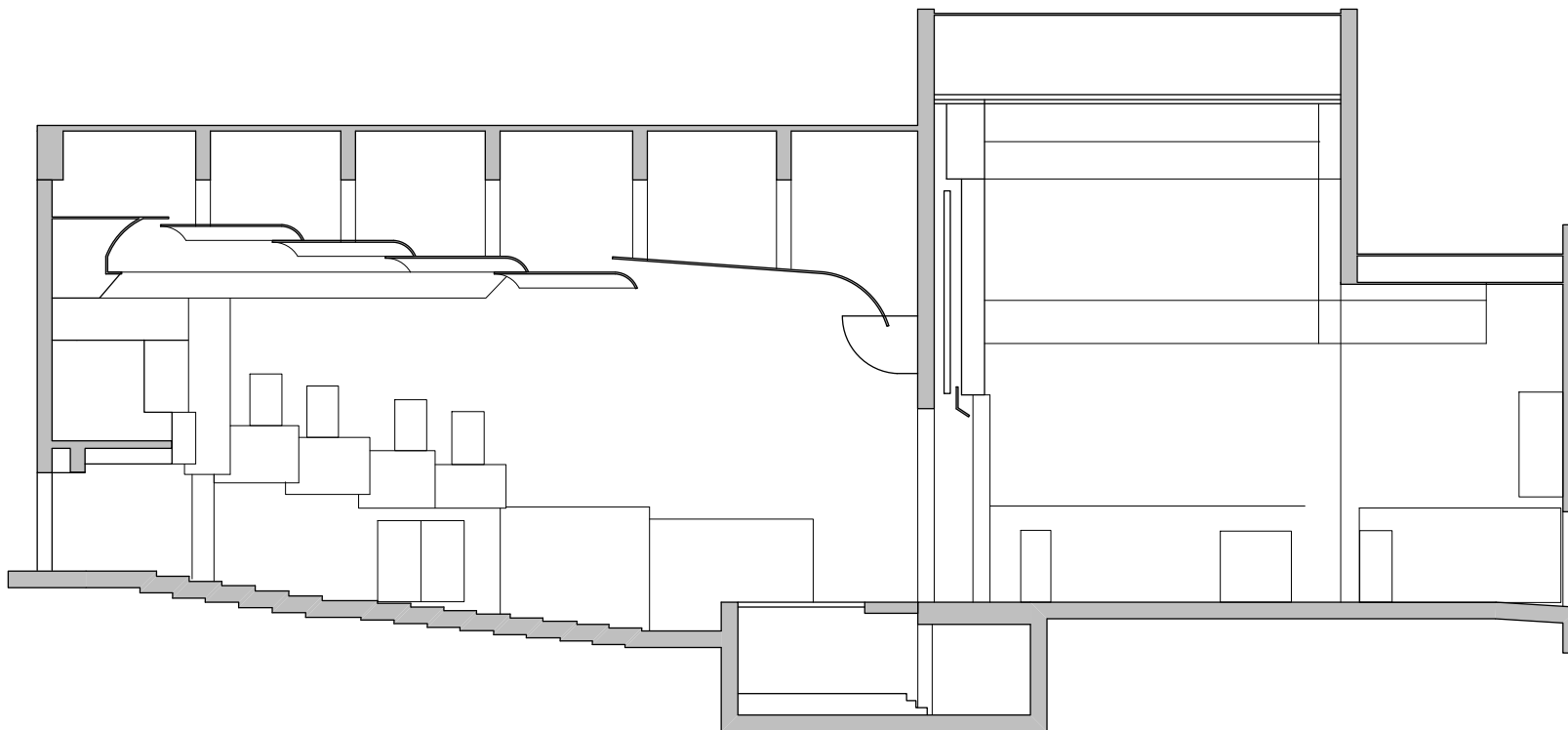
Madlenianum, Beograd presek R 1:200
