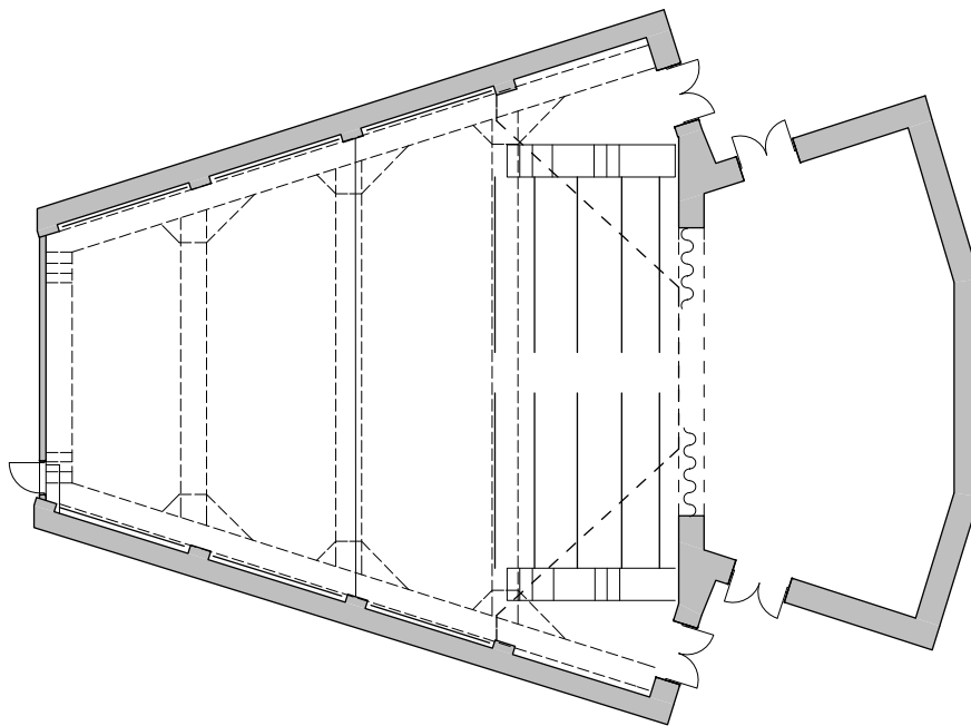
BITEF, Beograd osnova R 1:200
