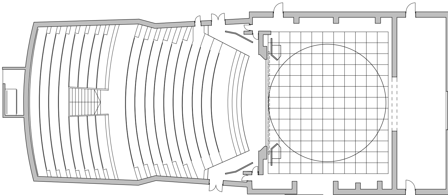
Beogradsko dramsko pozorište osnova velike sale R 1:200
