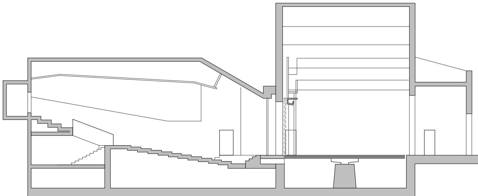
Beogradsko dramsko pozorište presek velike sale R 1:200
