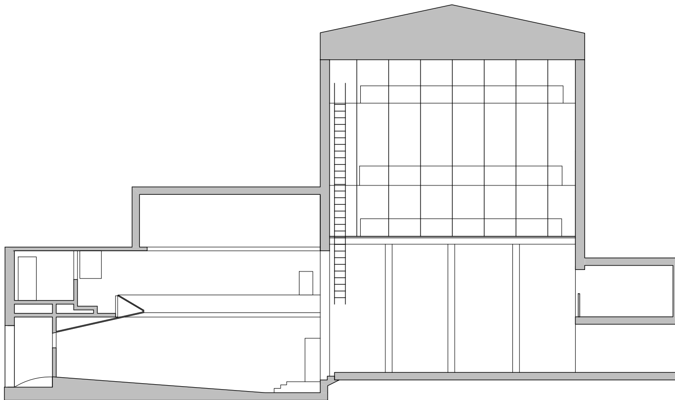
Atelje 212, Beograd presek R 1:200
