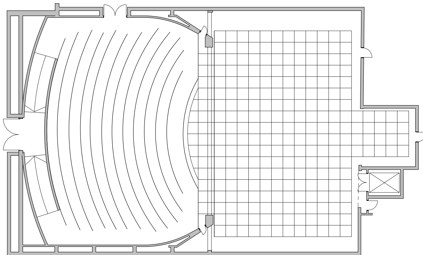
Atelje 212, Beograd osnova R 1:200
