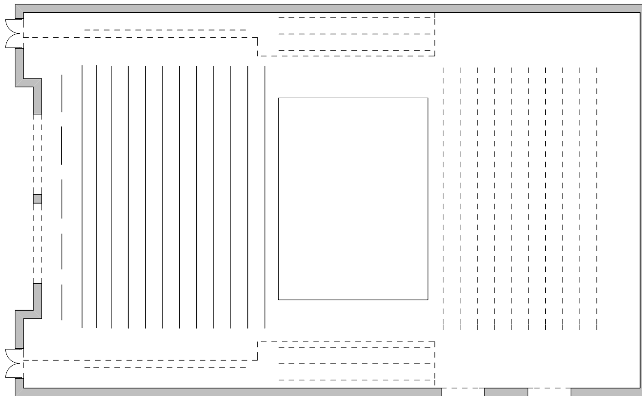
Zvezdara teatar, Beograd osnova velike sale R 1:200
