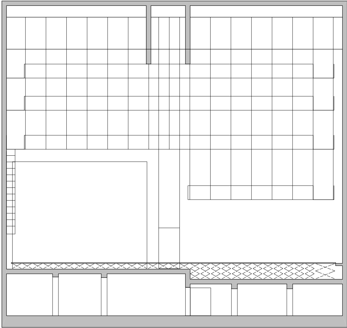
Narodno Pozorište u Subotici presek R 1:200
