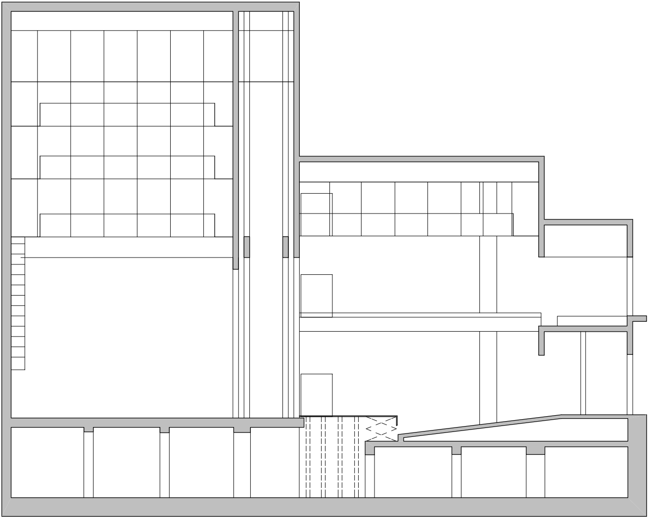
Narodno Pozorište u Subotici presek R 1:200
