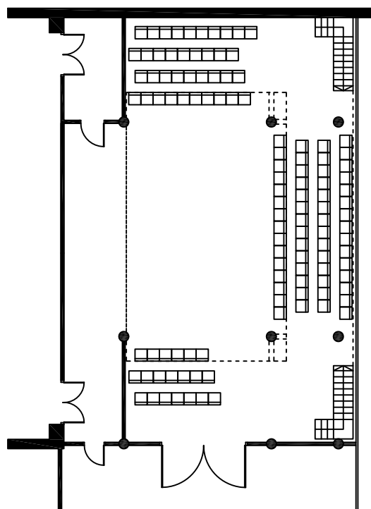
osnova partera
