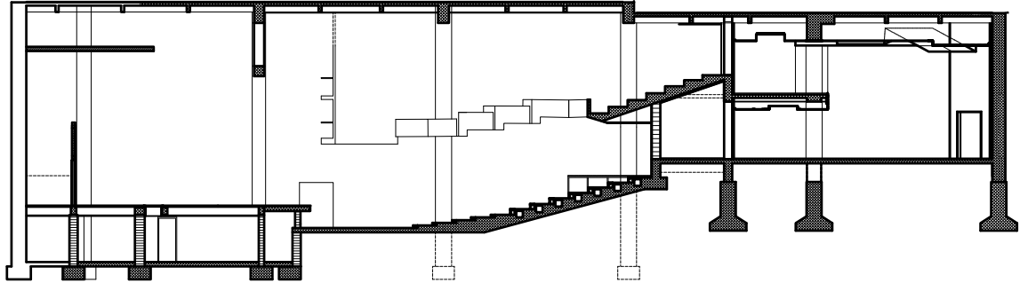
presek
