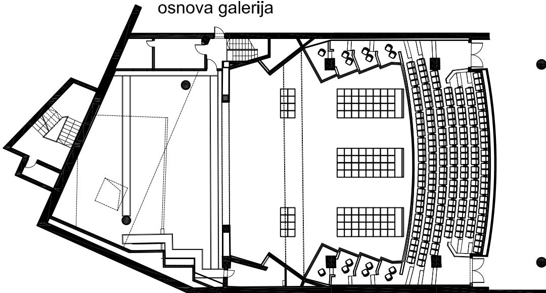
osnova partera
