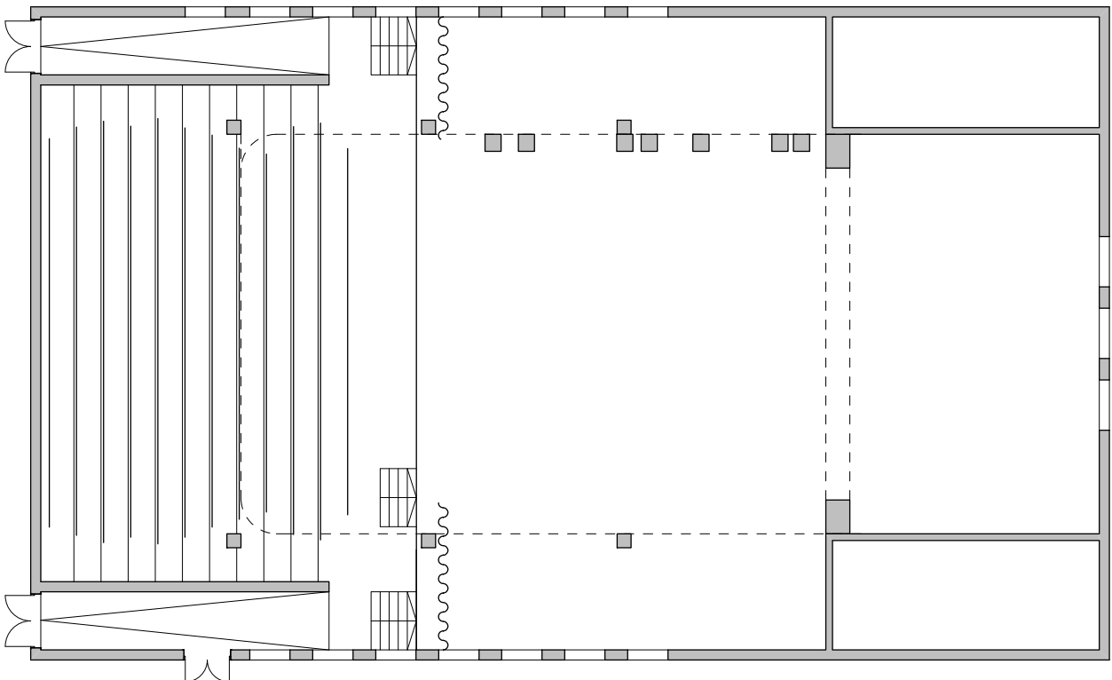
Narodno pozorište u Subotici osnova sale "Jadran" R 1:200
