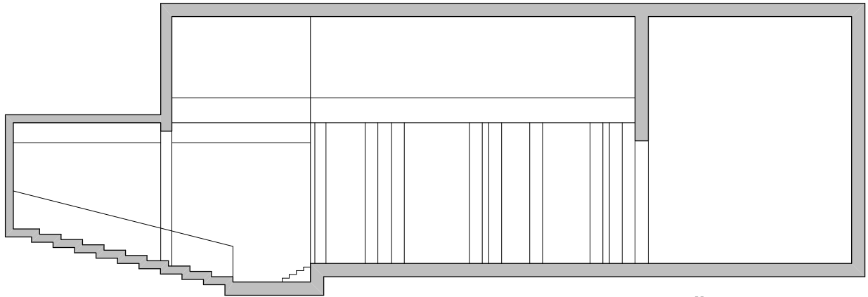
Narodno pozorište u Subotici presek kroz salu "Jadran" R 1:200
