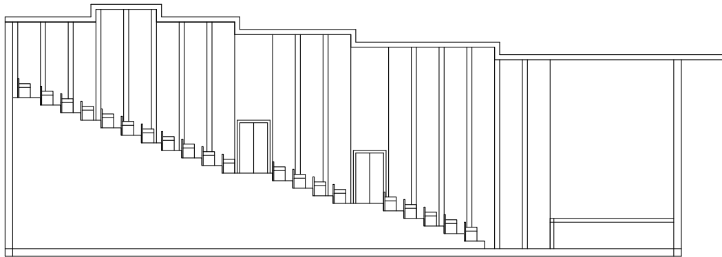
presek
