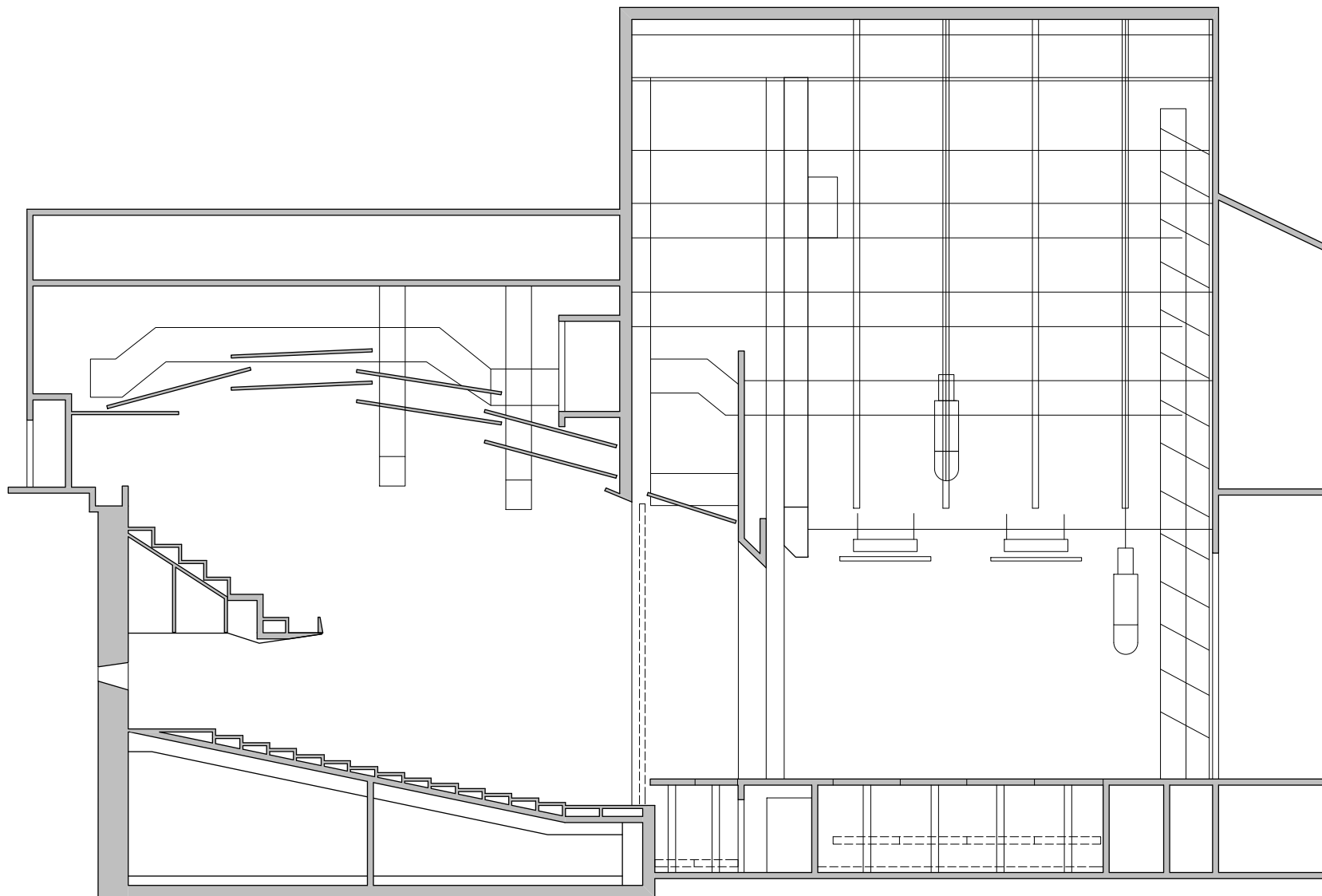
Jugoslovensko dramsko pozorište, Beograd presek velike sale R 1:200
