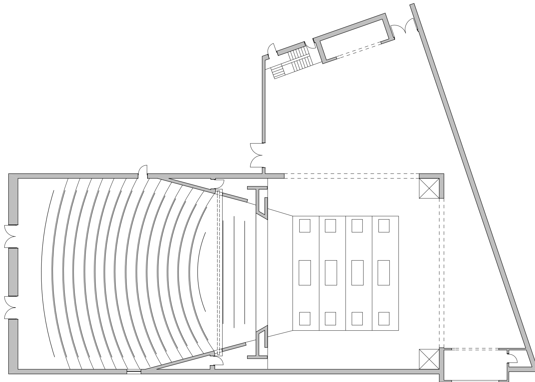
Jugoslovensko dramsko pozorište, Beograd osnova velike sale R 1:200
