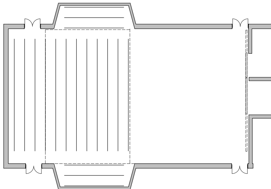
Narodno pozorište, Beograd Scena Raša Plaović R 1:200
