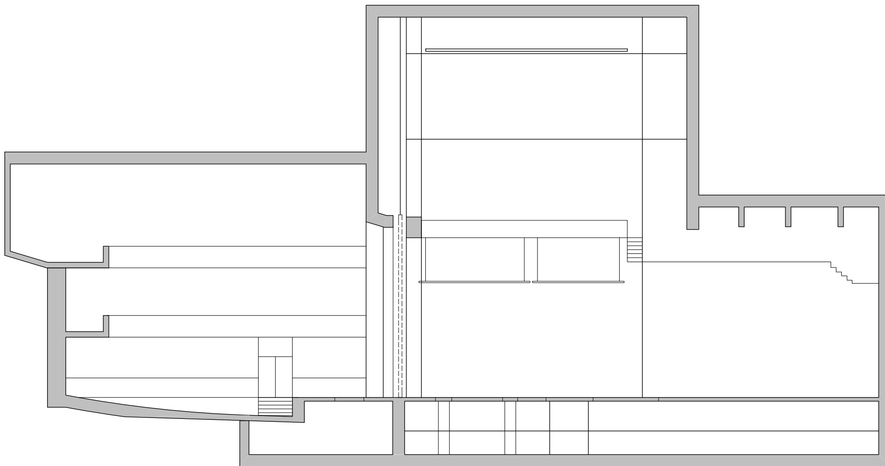
Narodno pozorište, Beograd presek velike sale R 1:200
