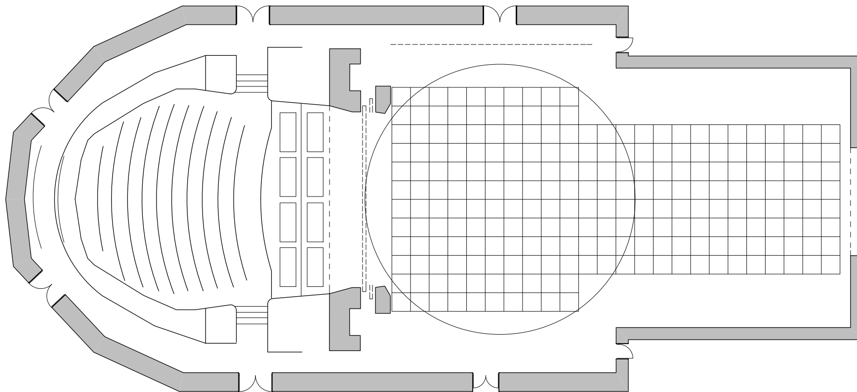
Narodno pozorište, Beograd osnova velike sale R 1:200
